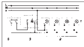
3. Conexão mediante comutador inversor para modo manual e automático
